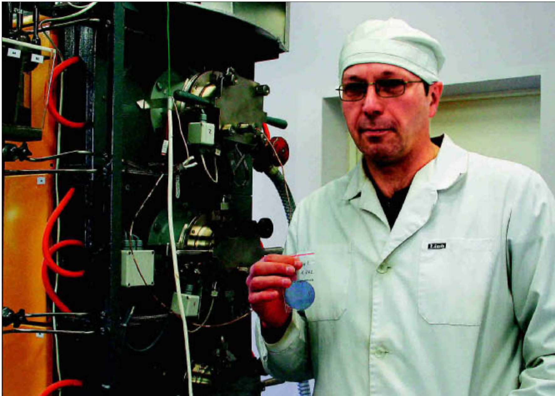
Tartu kõrgtehnoloogiafirma OÜ Clifton epitaksi tehnoloog Viktor Korsmik firma südames – seadmete juures, kus kasvatatakse pooljuhtkristalle. Korsmiku käes on kahetollise läbimõõduga pooljuhtkristall.
